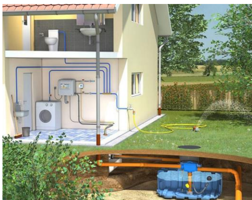
Systeem hergebruik regenwater in de woning
